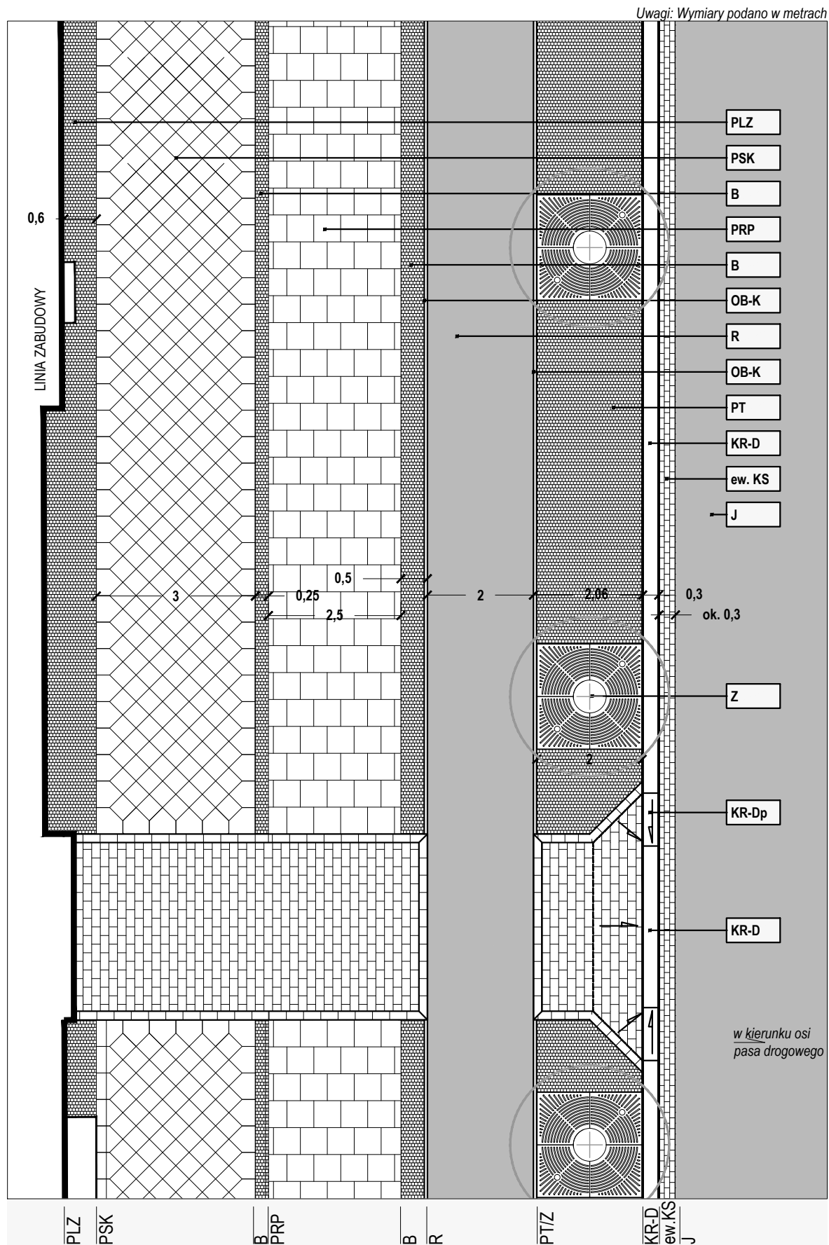
R y c. I/61 | Przykładowa teoretyczna sekwencja prosta dla ulicy o znacznej szerokości w l.rozgr. cz.1
