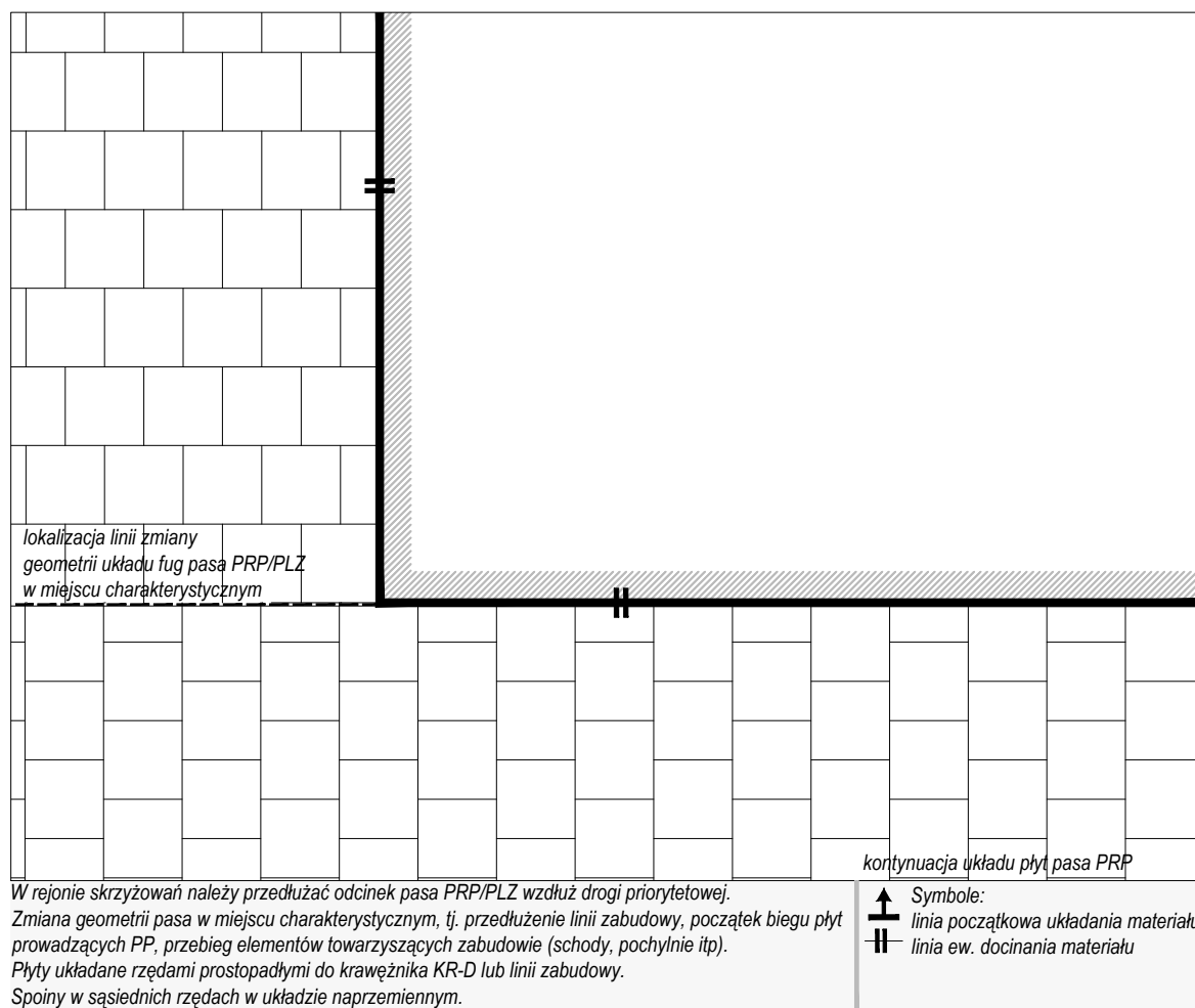
R y c. III/4 IPLZ - pas przylegający do linii zabudowy Zmiana przebiegu układu fug
