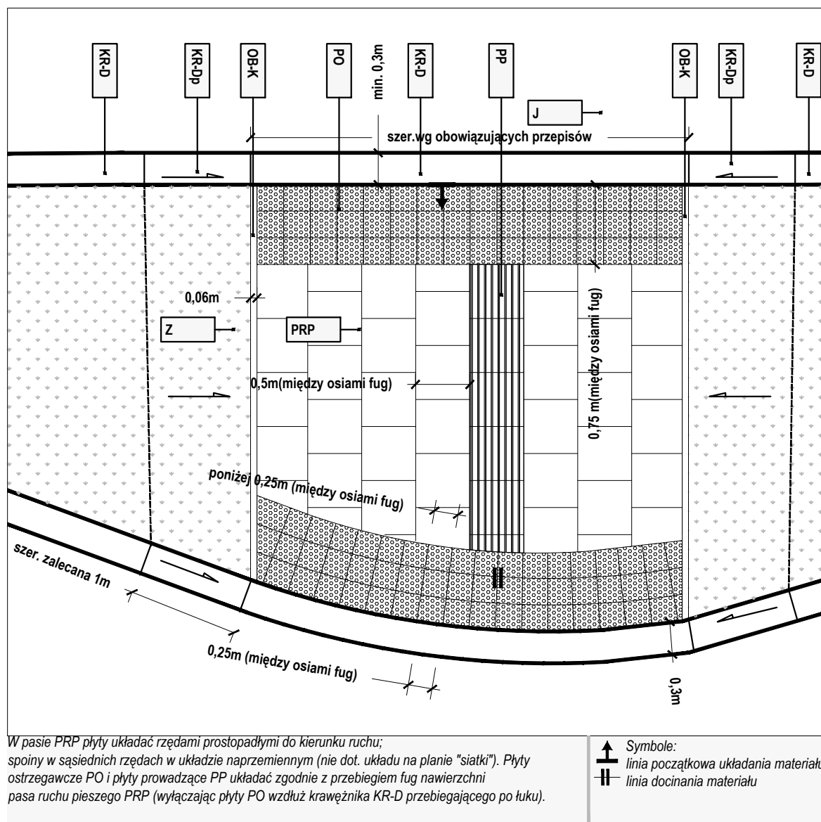
R y c. I/58 | Azyl dla pieszych
