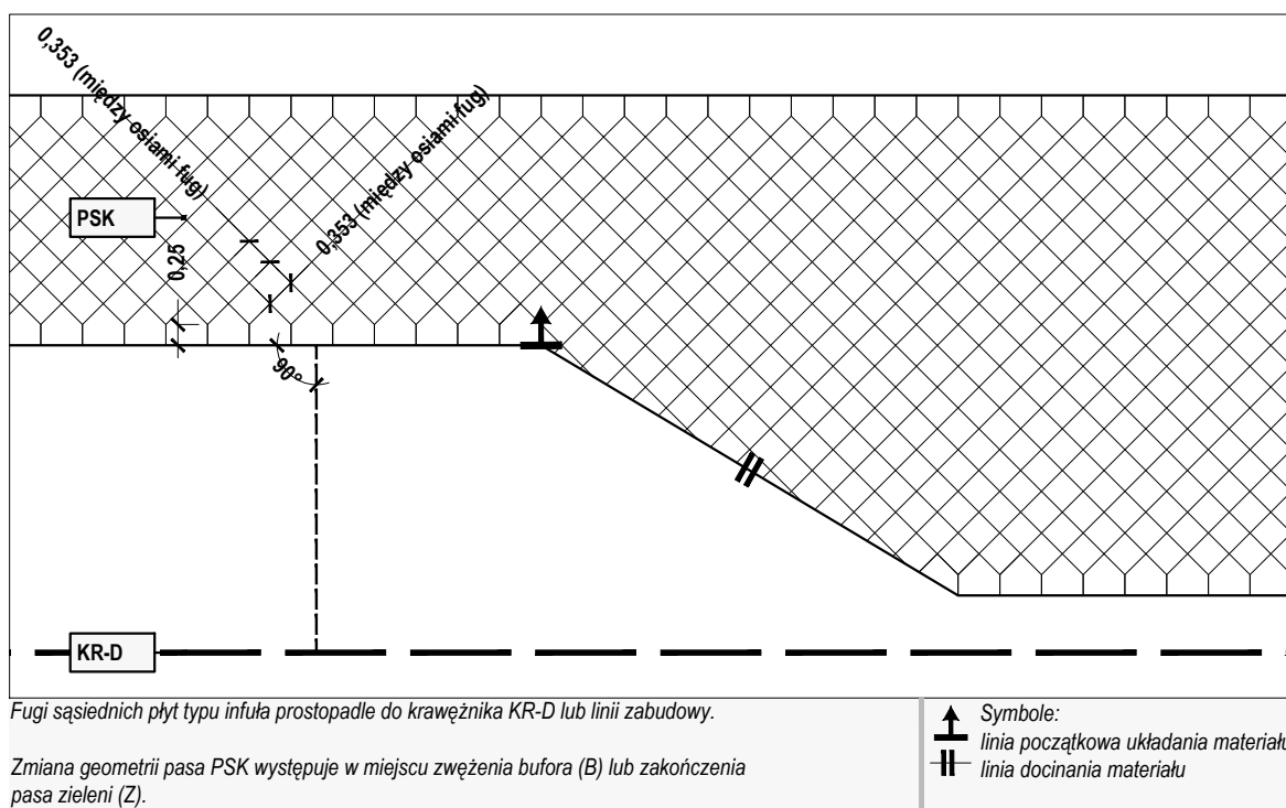
R y c. III/10 IPSK - pas społeczno-kulturowy
