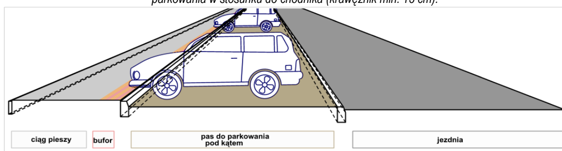
Rys.16. Ciąg pieszony prowadzony wzdłuż miejsc do parkowania zorganizowanego „pod kątem” – segregacja bez zróżnicowania wysokości nawierzchni miejsc do parkowania w stosunku do chodnika (krawężnik do 15 cm), ale z zastosowaniem bufora bezpieczeństwa.
