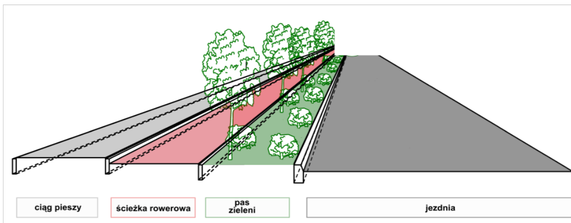
Rys.22. Ulica z drogą dla rowerów przylegającą do ciągu pieszego z oddzieleniem od jezdni pasem zieleni (ciąg pieszey i rowerowy różnicowane wysokością i rodzajem nawierzchni).
