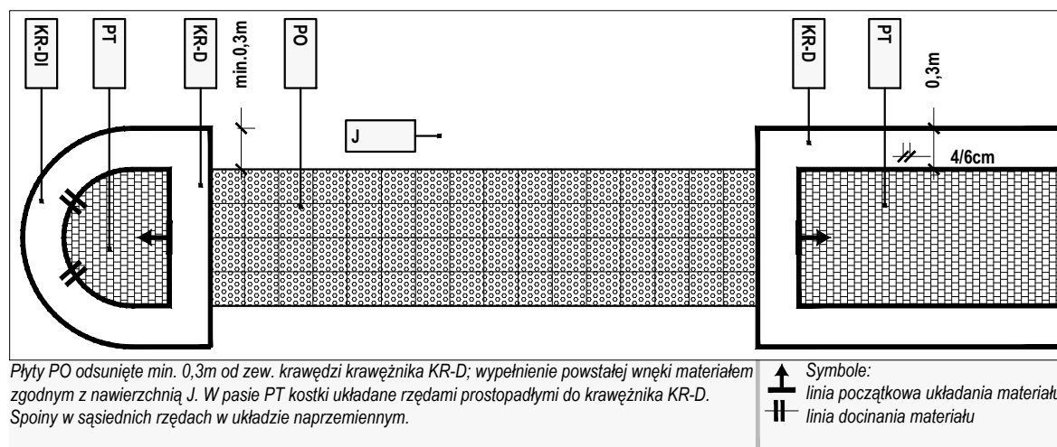
R y c. I/59 | Azyl dla pieszych
