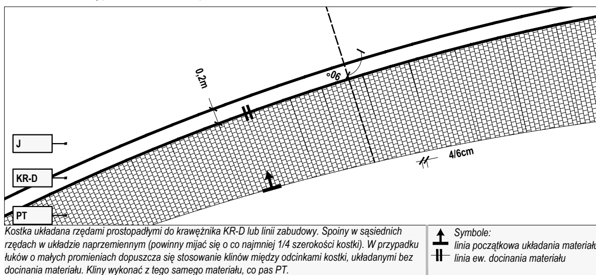
R y c. II/21 IPT - pas techniczny Przebieg po łuku, zmienna szerokość pasa PT
