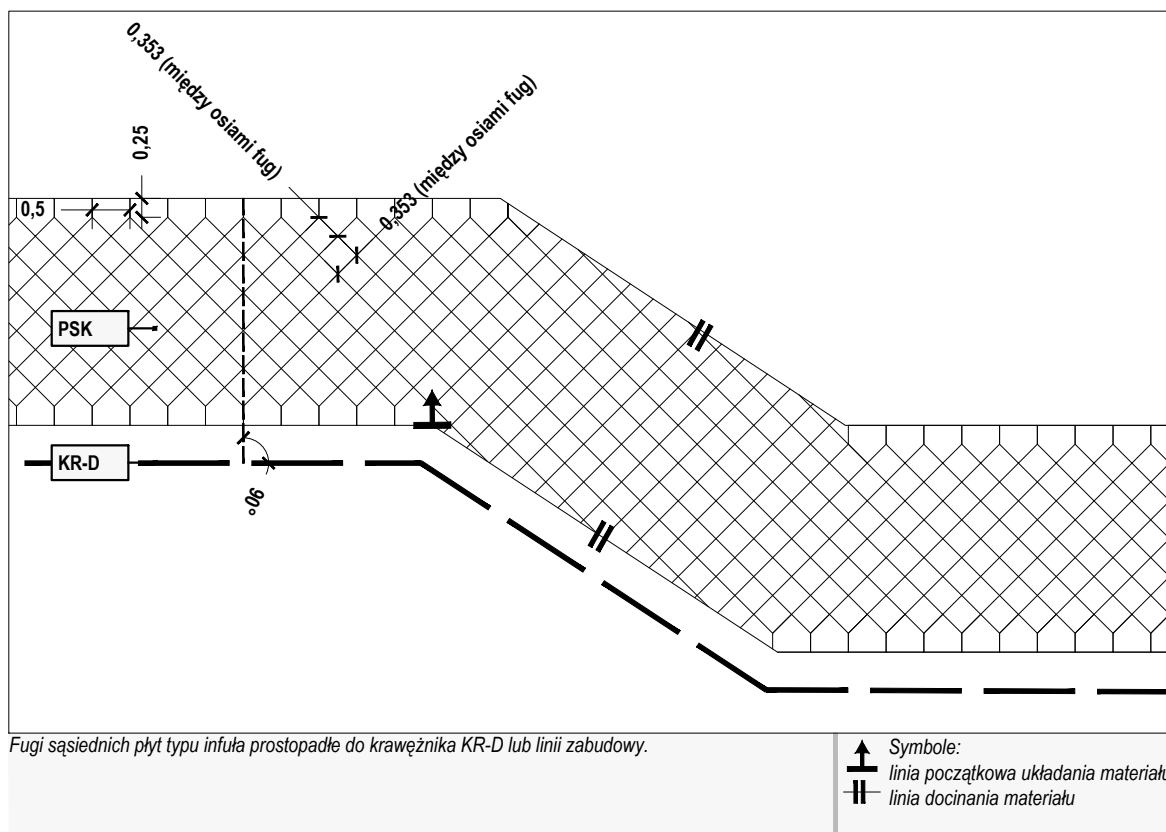
R y c. III/9 IPSK - pas społeczno-kulturowy
