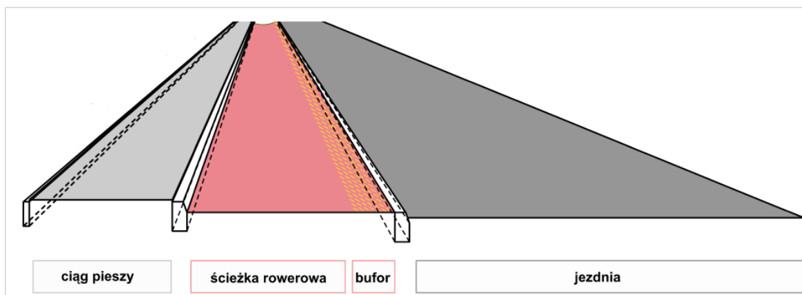
Rys.23. Ulica z drogą dla rowerów oddzieloną od jezdni buforem bezpieczeństwa (ciąg pieszey i rowerowy różnicowane wysokością i rodzajem nawierzchni).
