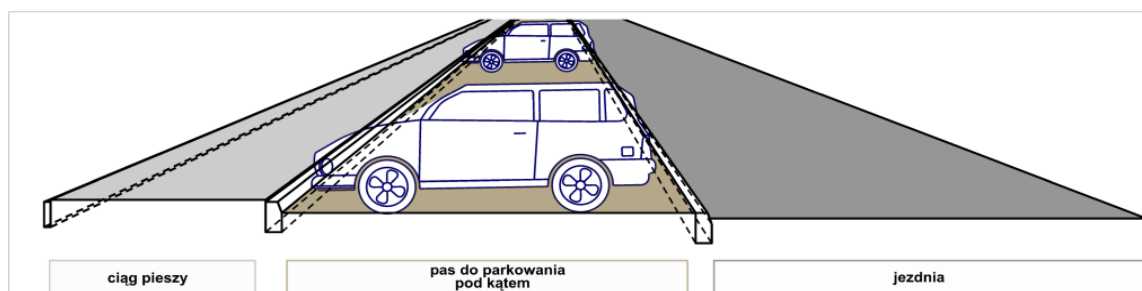
Rys.15. Ciąg pieszony prowadzony wzdłuż miejsc do parkowania zorganizowanych „pod kątem” – segregacja w postaci zróżnicowanej wysokości nawierzchni miejsc do parkowania w stosunku do chodnika (krawężnik min. 15 cm).
