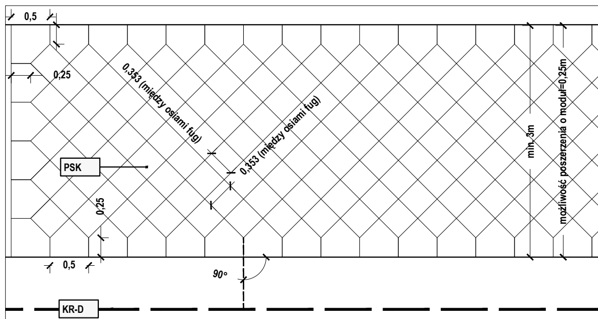
R y c. I/5 |PSK - pas społeczno-kulturowy
