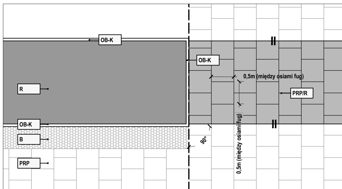
R y c. II/34 | R - droga rowerowa poza jezdnią, w strefie ciągu pieszego Typowy sposób wydzielenia drogi rowerowej R w rejonie skrzyżowań.
